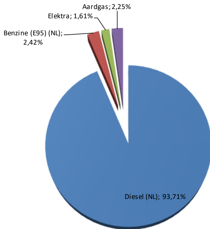
CO2 Footprint 2023
